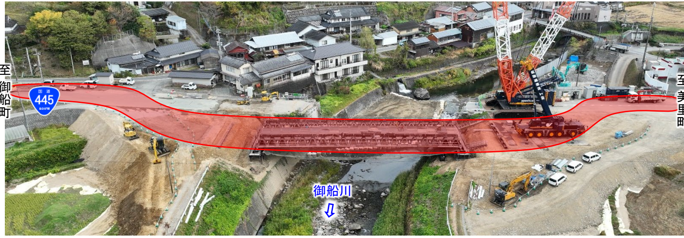
仮設道路イメージ
