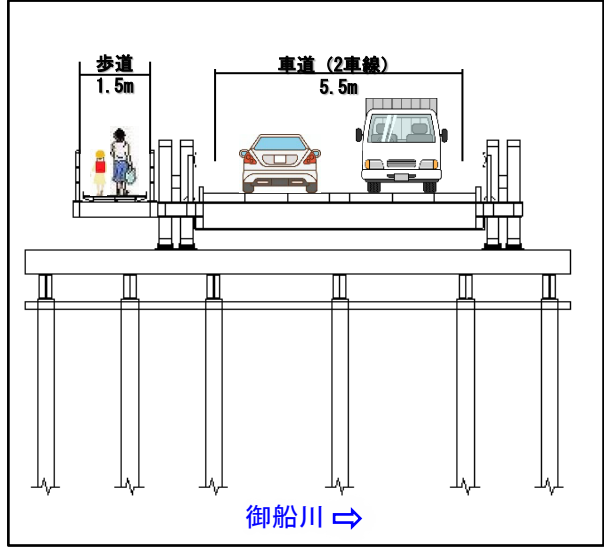
応急組立橋断面図
