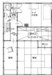
2階平面図
